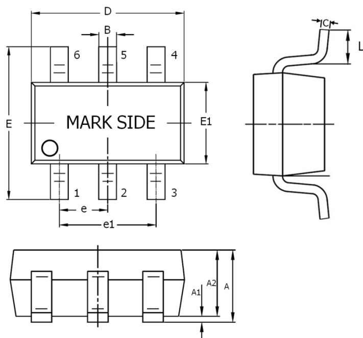
TSOT-23-6L Package (Unit: mm)
