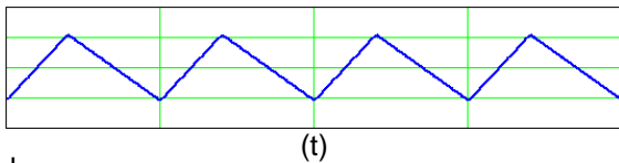
V_{\text{RIPPLE(ESR)}}(t)
