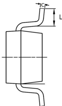
TSOT-23-5L Package (Unit: mm)
