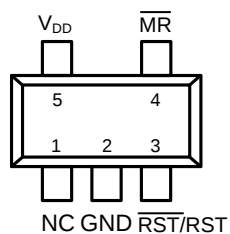
S8 Package (TSOT-23-5)
