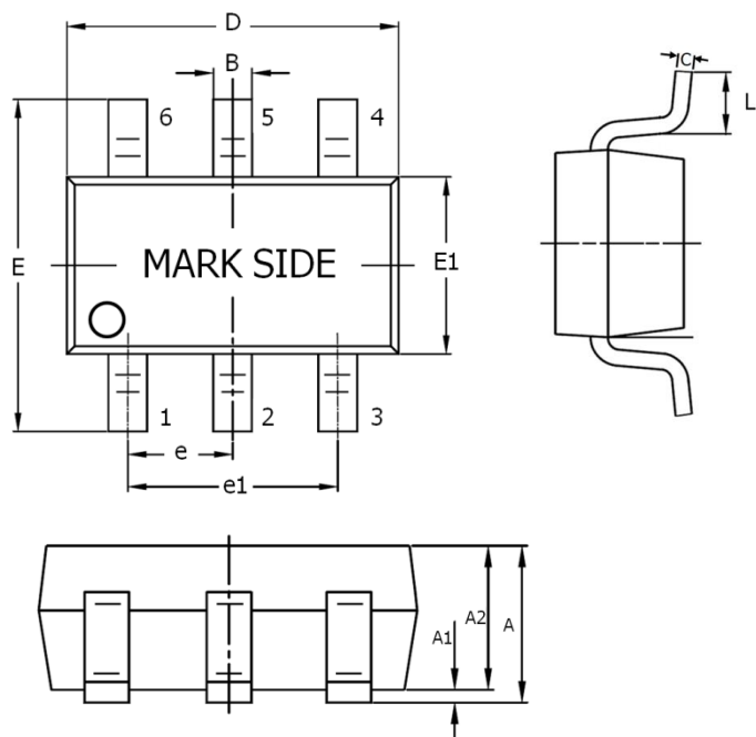
TSOT-23-6L Package (Unit: mm)
